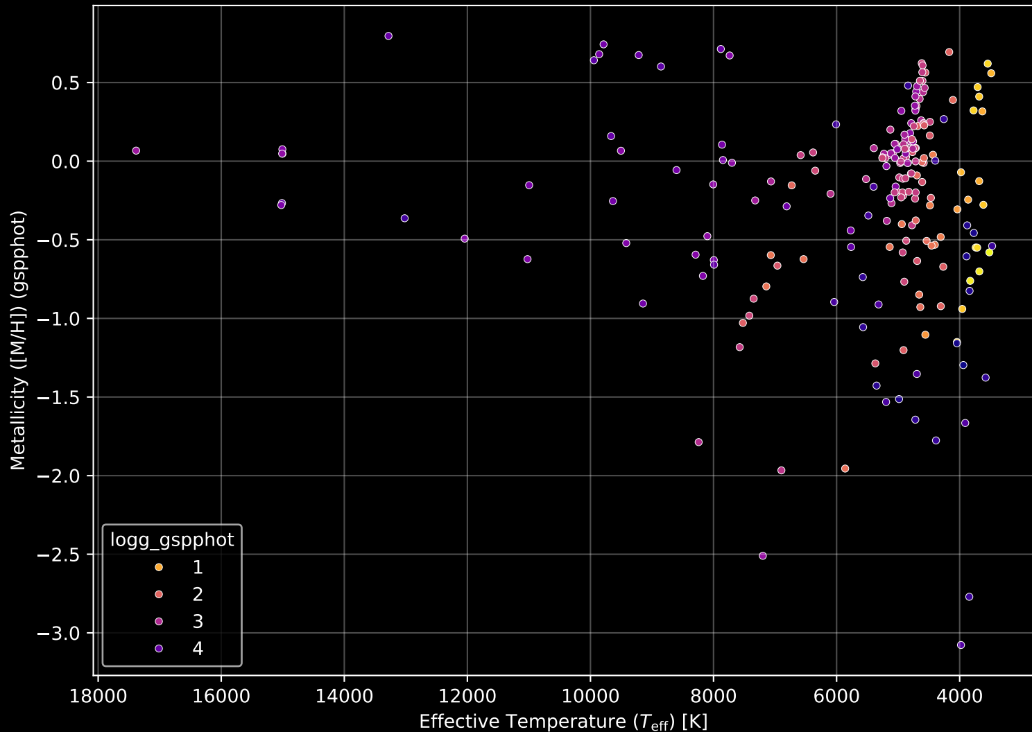
APOGEE DR17 Field: [340+00] Stellar Population Parameters (n= 209)
